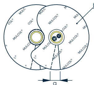
a: Überlappung, mindestens 10 mm b: Multidisc
