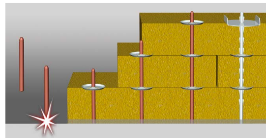
Befestigung mit Schweiß-Stiften
