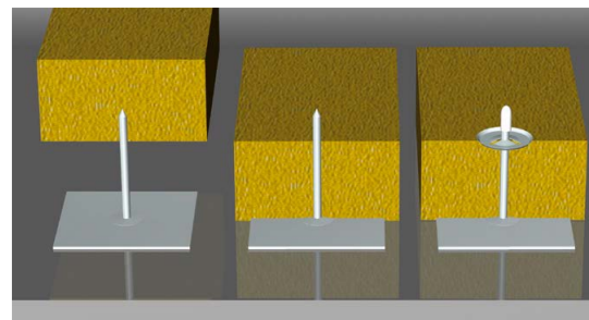
Selbstklebende Befestigung mit CLAVU-fix
