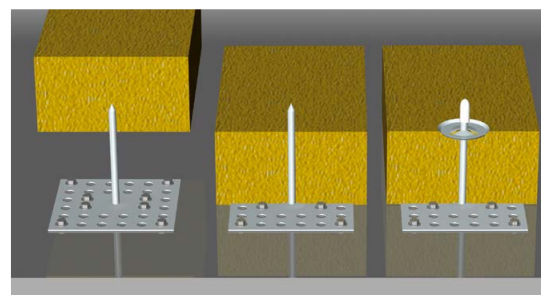
Schraub- bzw. Niet-Befestigung mit CLAVU-por
