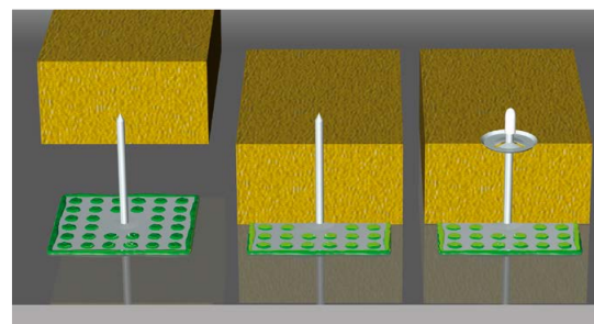
Klebe-Befestigung mit CLAVU-por
