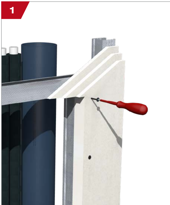
1 Umlaufend Montageprofile befestigen. (bündig mit der Wandöffnung)
