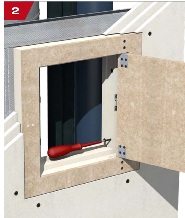
2 Brandverschlussdeckel entfernen und Einbaurahmen an den Montageprofilen befestigen.
