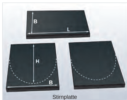
Stirnplatte
