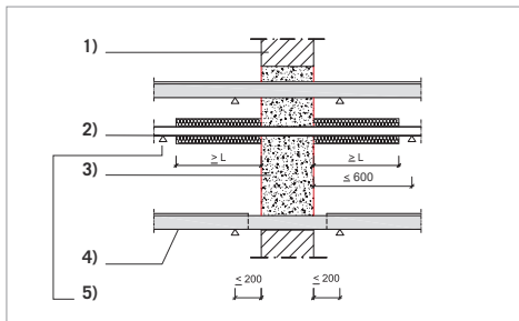
Bild 1: Unterstützung von Rohren und Kabel / Kabeltragekonstruktionen in Wänden
